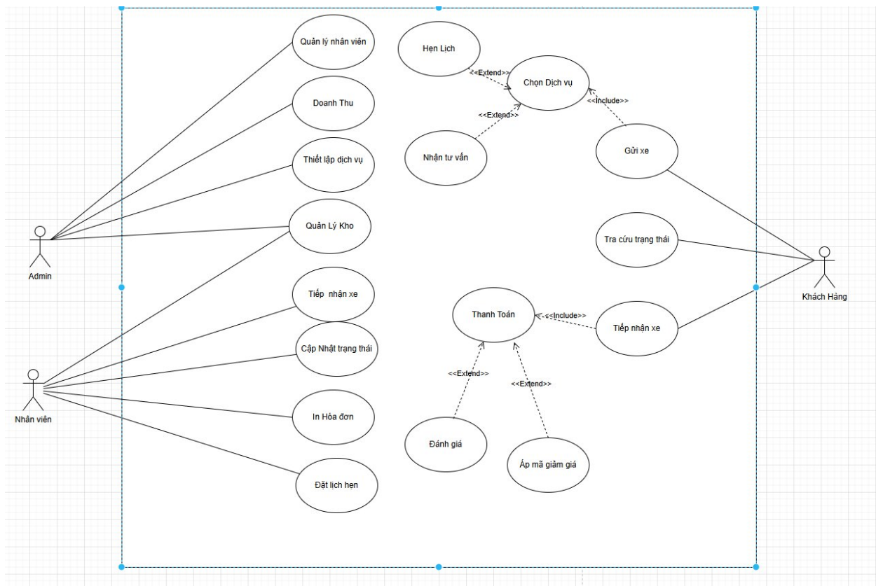
Sơ đồ USE CASE tổng quát
